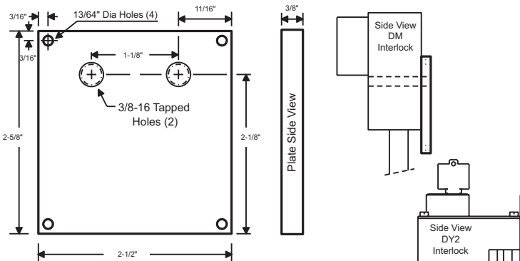
Optional DM2 Adapter Plate
